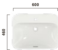
L5616CE Möbelwaschtisch LF 600mm, mit Hahnloch, mit Überlauf Furniture washbasin LF 600mm, with tap hole, with overflow
